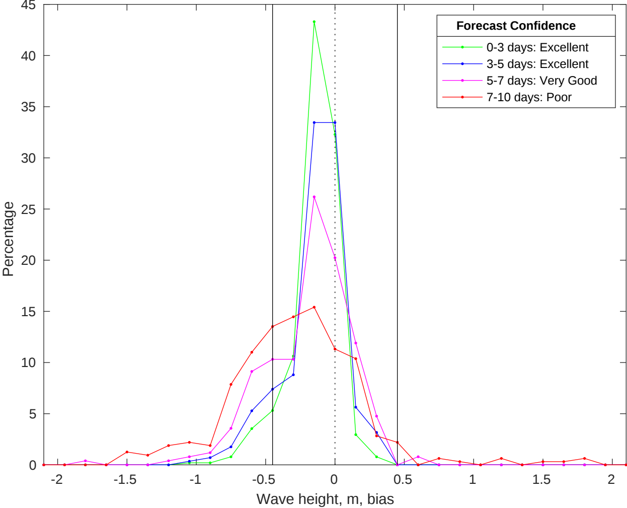
NDBC 42036 vs CMEMS Waves Bias Histogram: 15-Jan-2026
