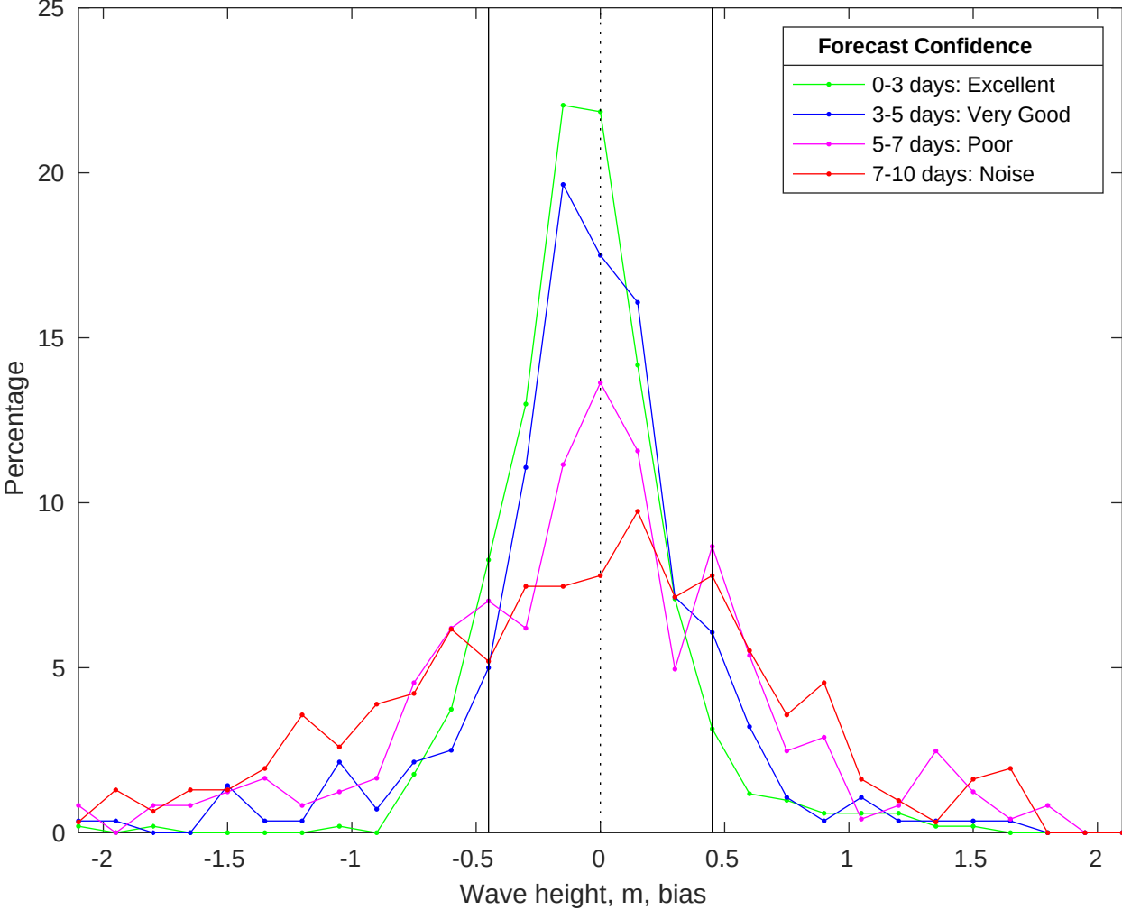
NDBC 44008 vs CMEMS Waves Bias Histogram: 15-Jan-2026
