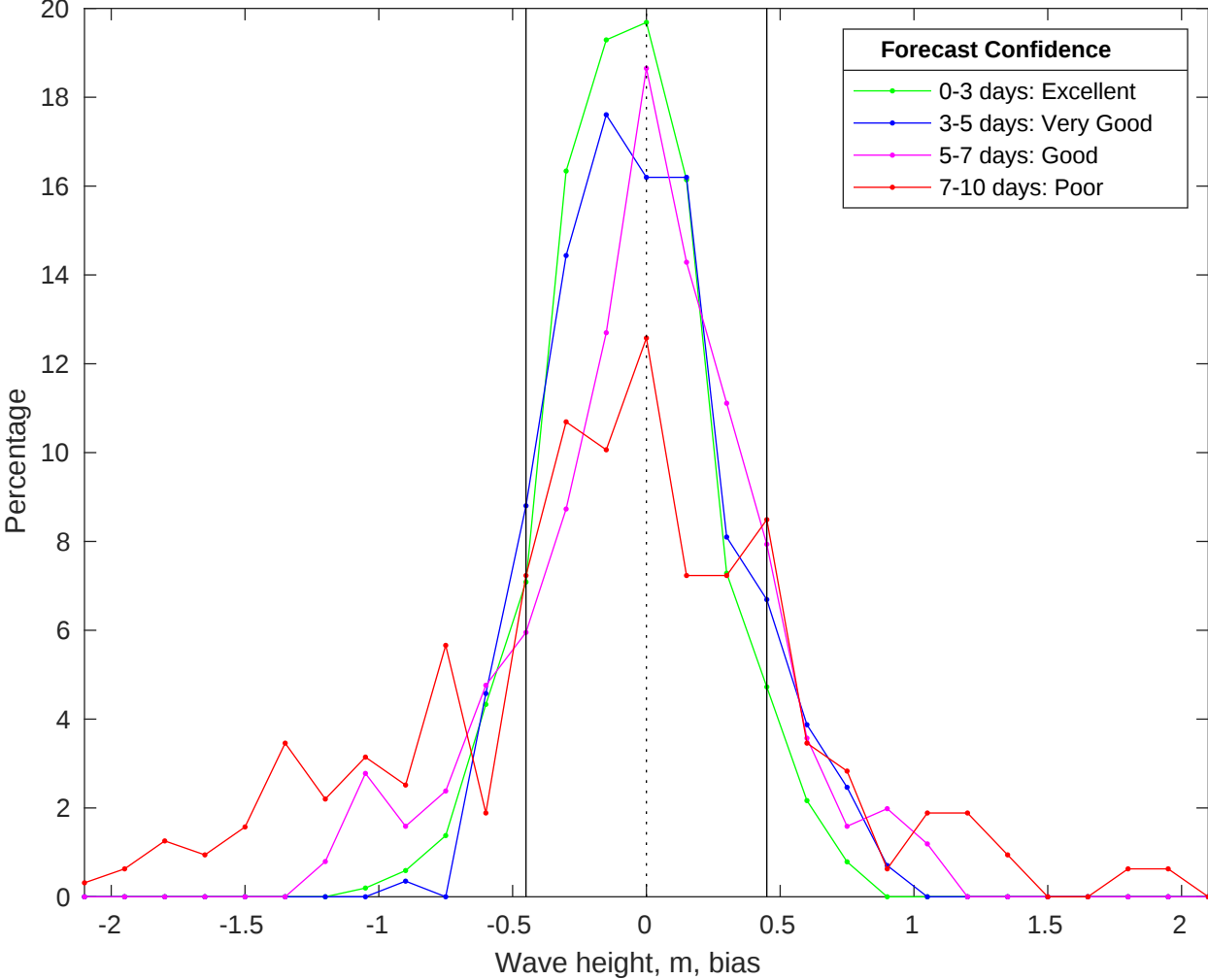
NDBC 46054 vs CMEMS Waves Bias Histogram: 15-Jan-2026
