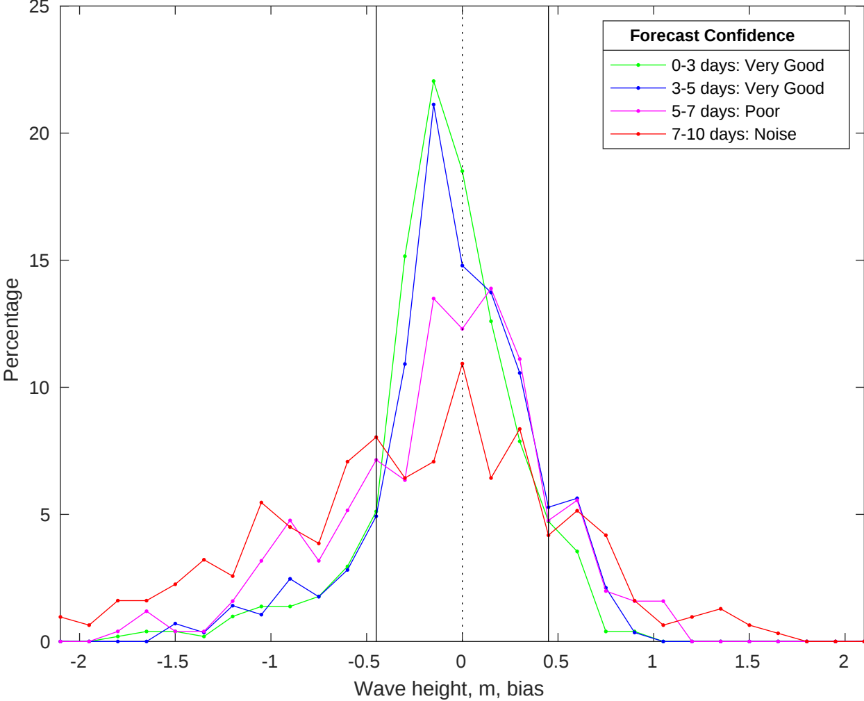
NDBC 46259 vs CMEMS Waves Bias Histogram: 15-Jan-2026
