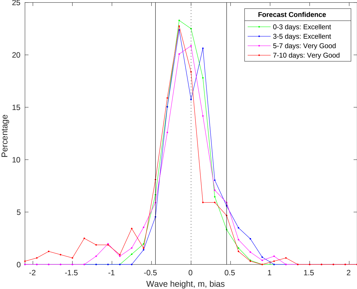
NDBC 46054 vs CMEMS Waves Bias Histogram: 19-Jan-2026
