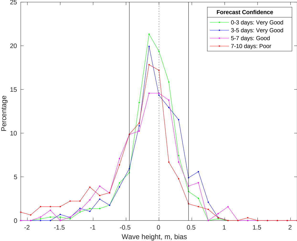
NDBC 46259 vs CMEMS Waves Bias Histogram: 19-Jan-2026
