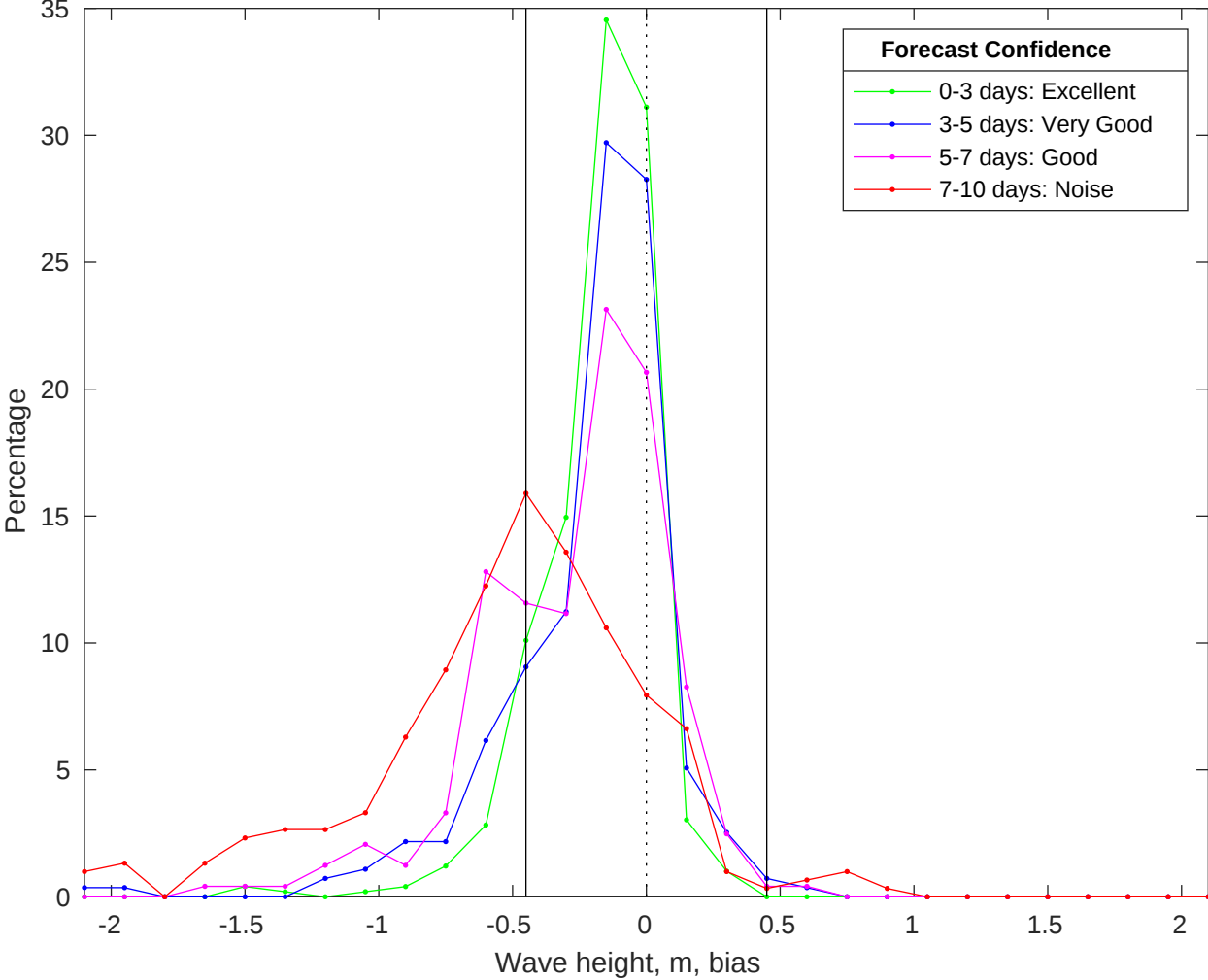
NDBC 42036 vs CMEMS Waves Bias Histogram: 20-Jan-2026
