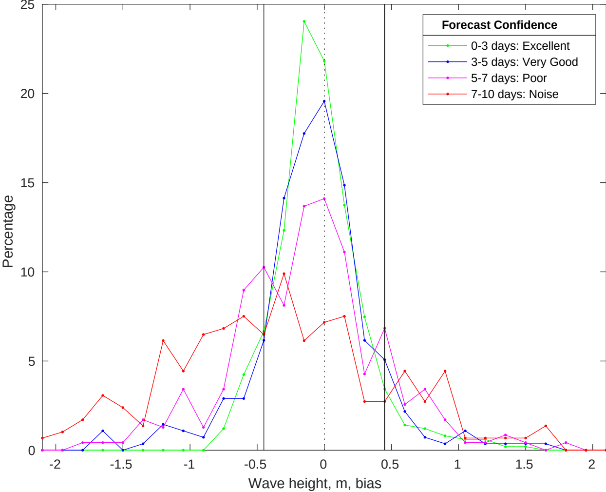
NDBC 44008 vs CMEMS Waves Bias Histogram: 20-Jan-2026
