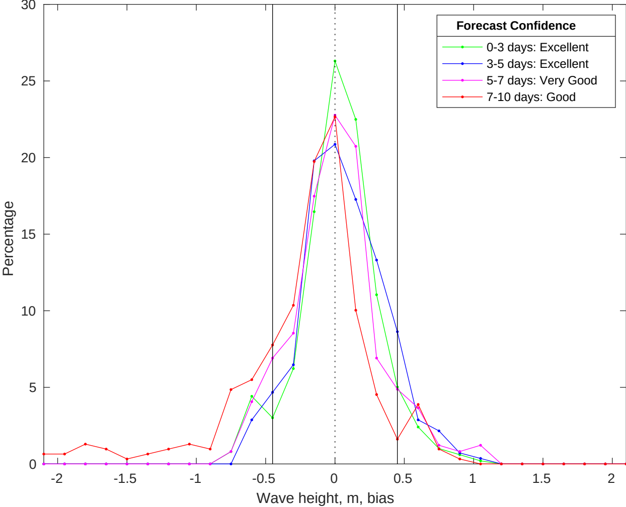
NDBC 46028 vs CMEMS Waves Bias Histogram: 20-Jan-2026
