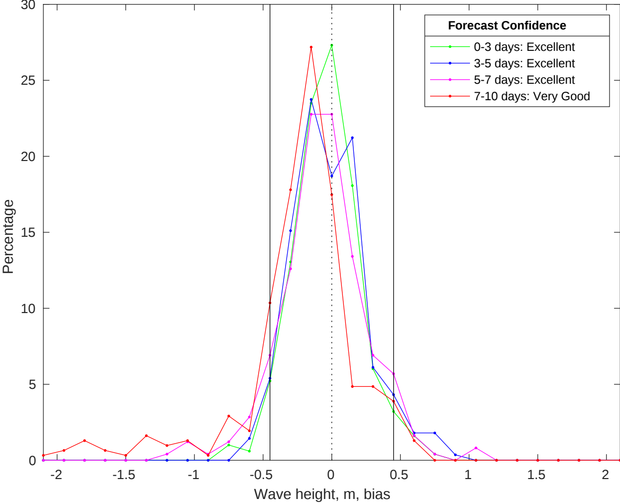
NDBC 46054 vs CMEMS Waves Bias Histogram: 20-Jan-2026
