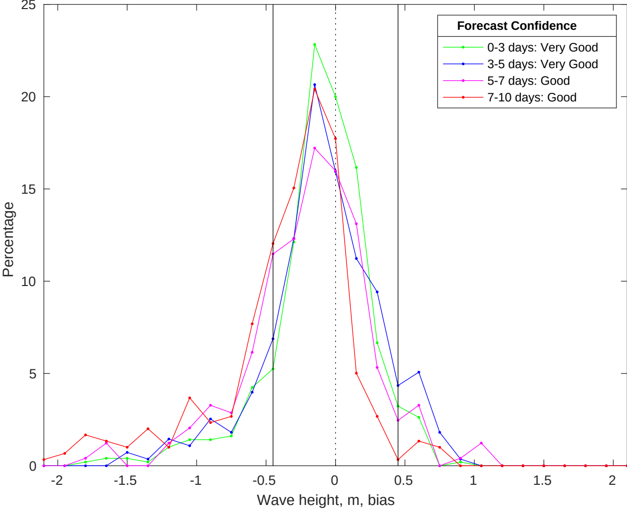
NDBC 46259 vs CMEMS Waves Bias Histogram: 20-Jan-2026
