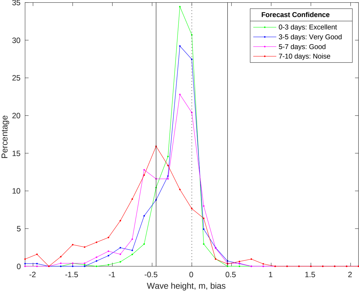
NDBC 42036 vs CMEMS Waves Bias Histogram: 21-Jan-2026
