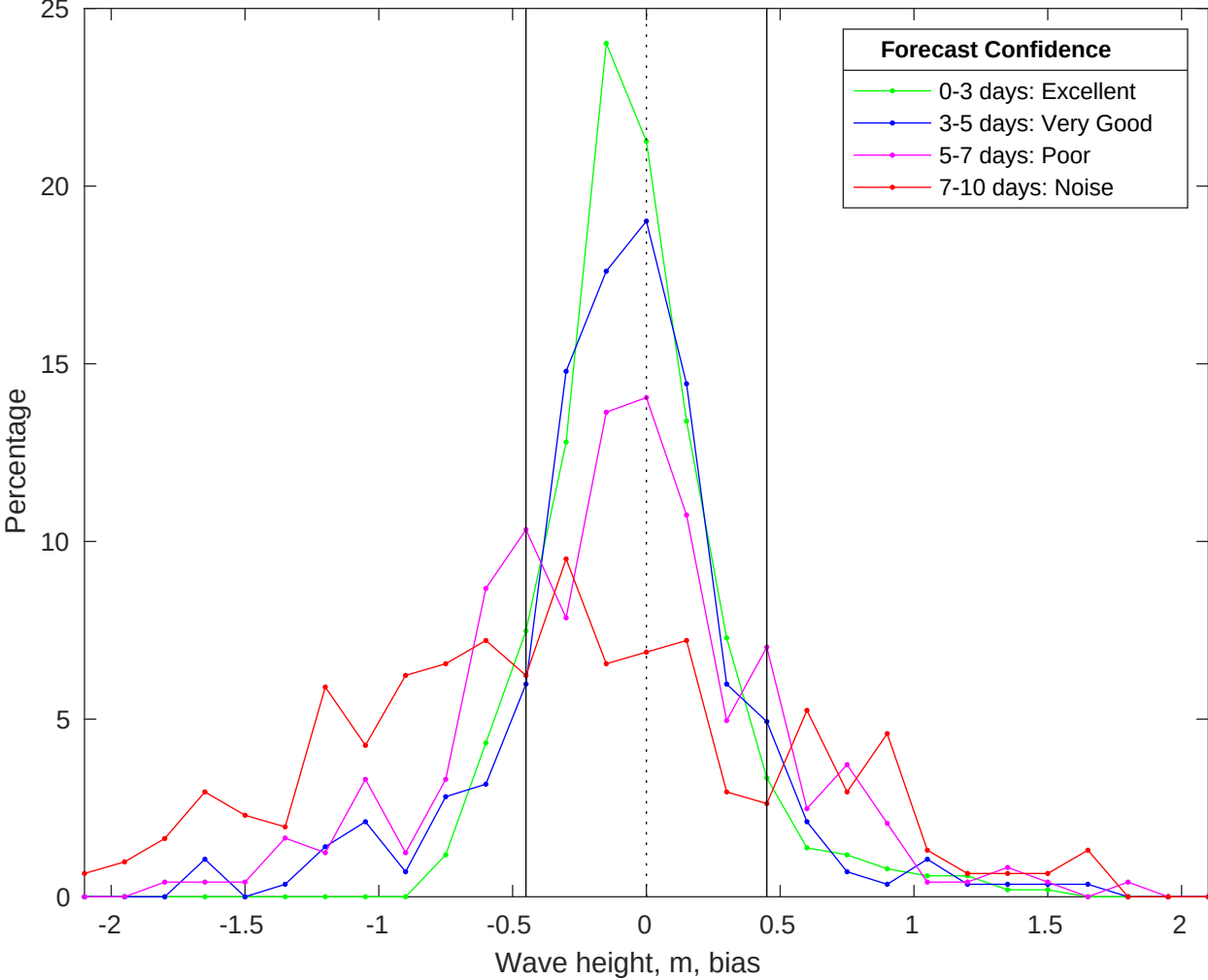
NDBC 44008 vs CMEMS Waves Bias Histogram: 21-Jan-2026
