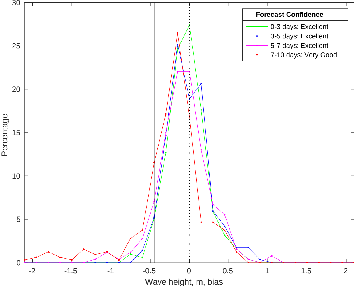
NDBC 46054 vs CMEMS Waves Bias Histogram: 21-Jan-2026
