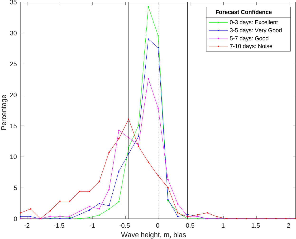
NDBC 42036 vs CMEMS Waves Bias Histogram: 22-Jan-2026
