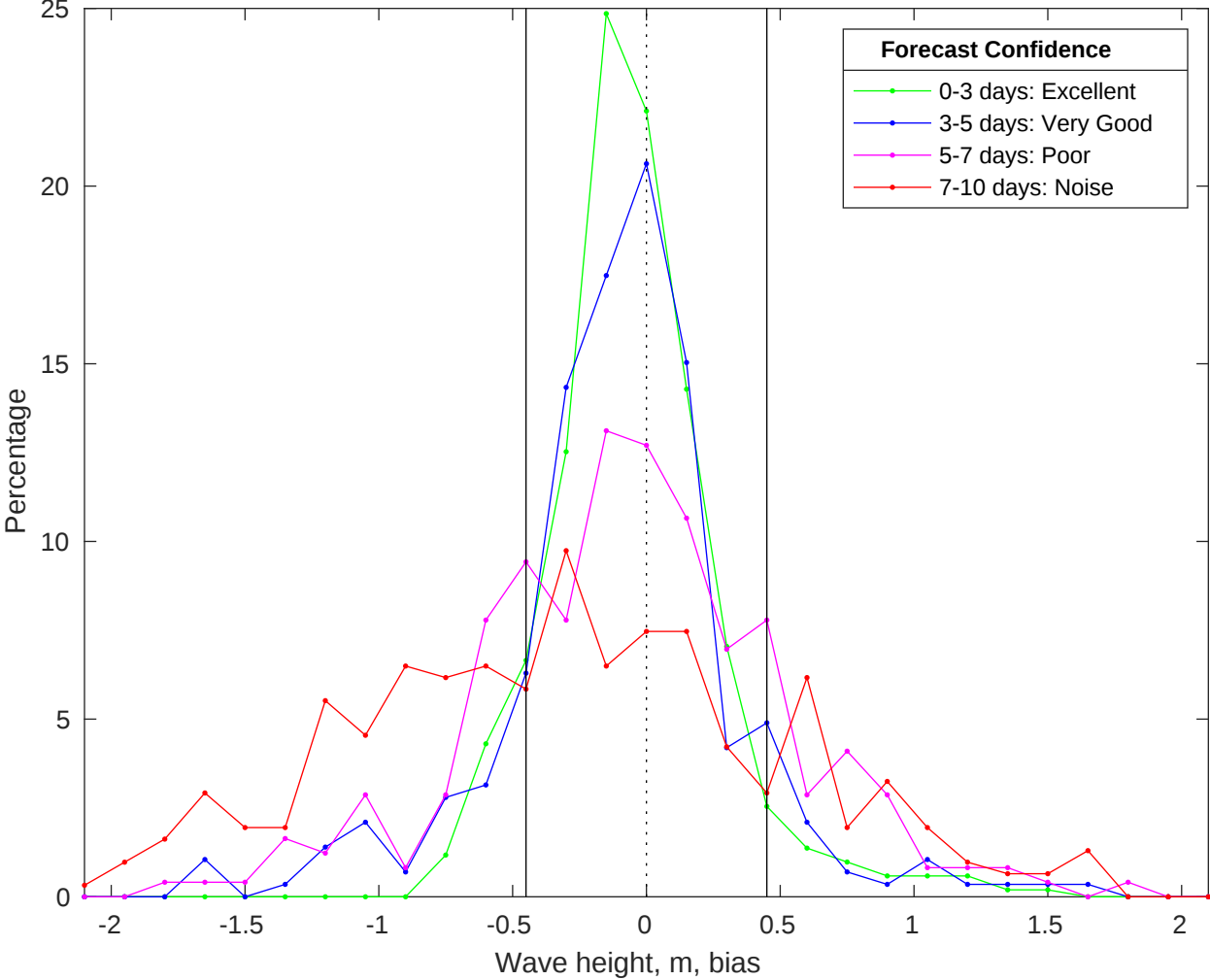
NDBC 44008 vs CMEMS Waves Bias Histogram: 22-Jan-2026
