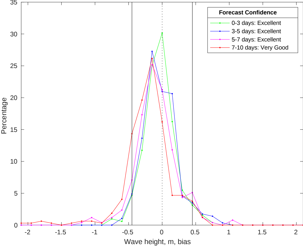
NDBC 46054 vs CMEMS Waves Bias Histogram: 22-Jan-2026
