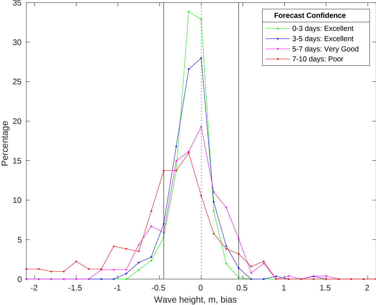
NDBC 41013 vs CMEMS Waves Bias Histogram: 25-Jan-2026
