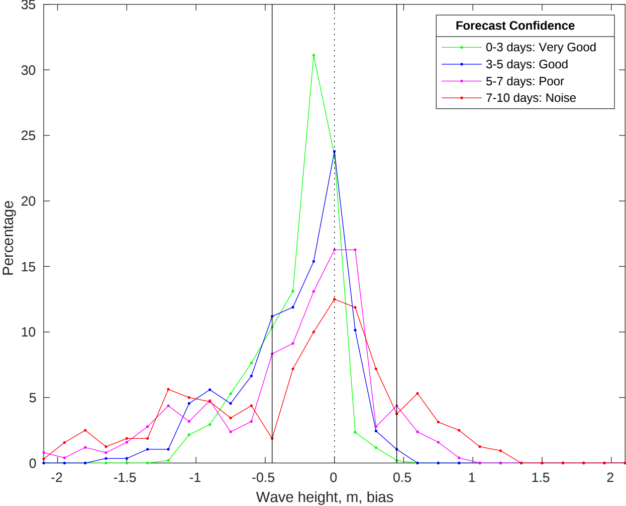
NDBC 42019 vs CMEMS Waves Bias Histogram: 25-Jan-2026
