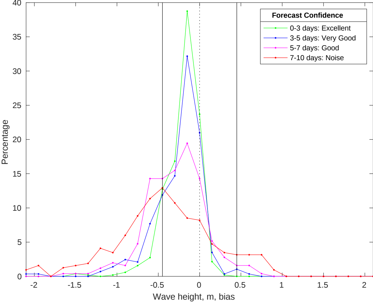
NDBC 42036 vs CMEMS Waves Bias Histogram: 25-Jan-2026
