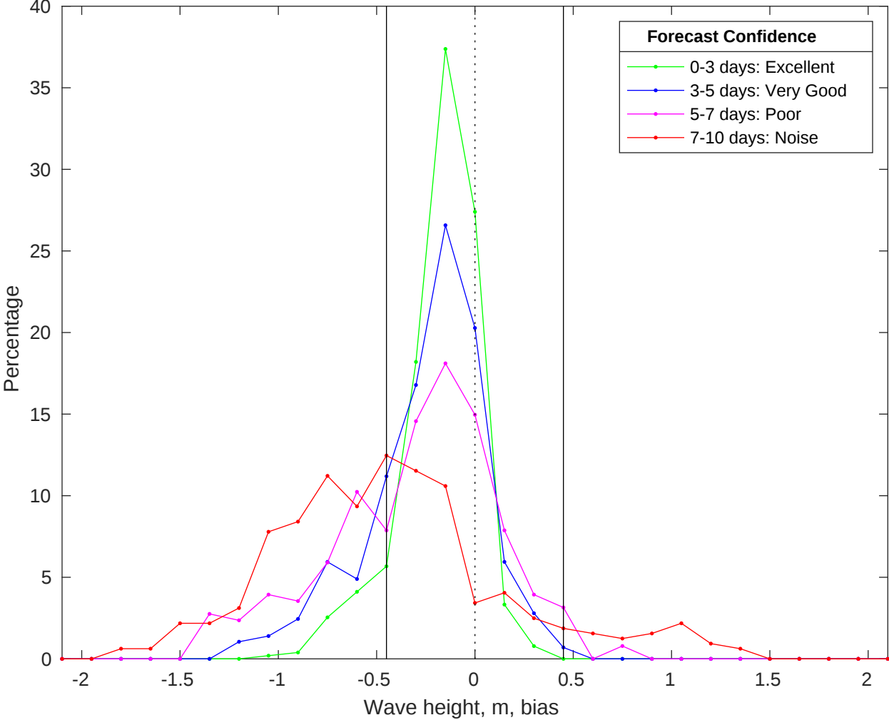
NDBC 42040 vs CMEMS Waves Bias Histogram: 25-Jan-2026
