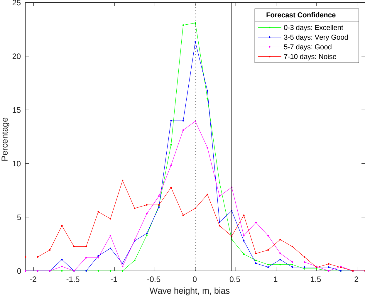
NDBC 44008 vs CMEMS Waves Bias Histogram: 25-Jan-2026
