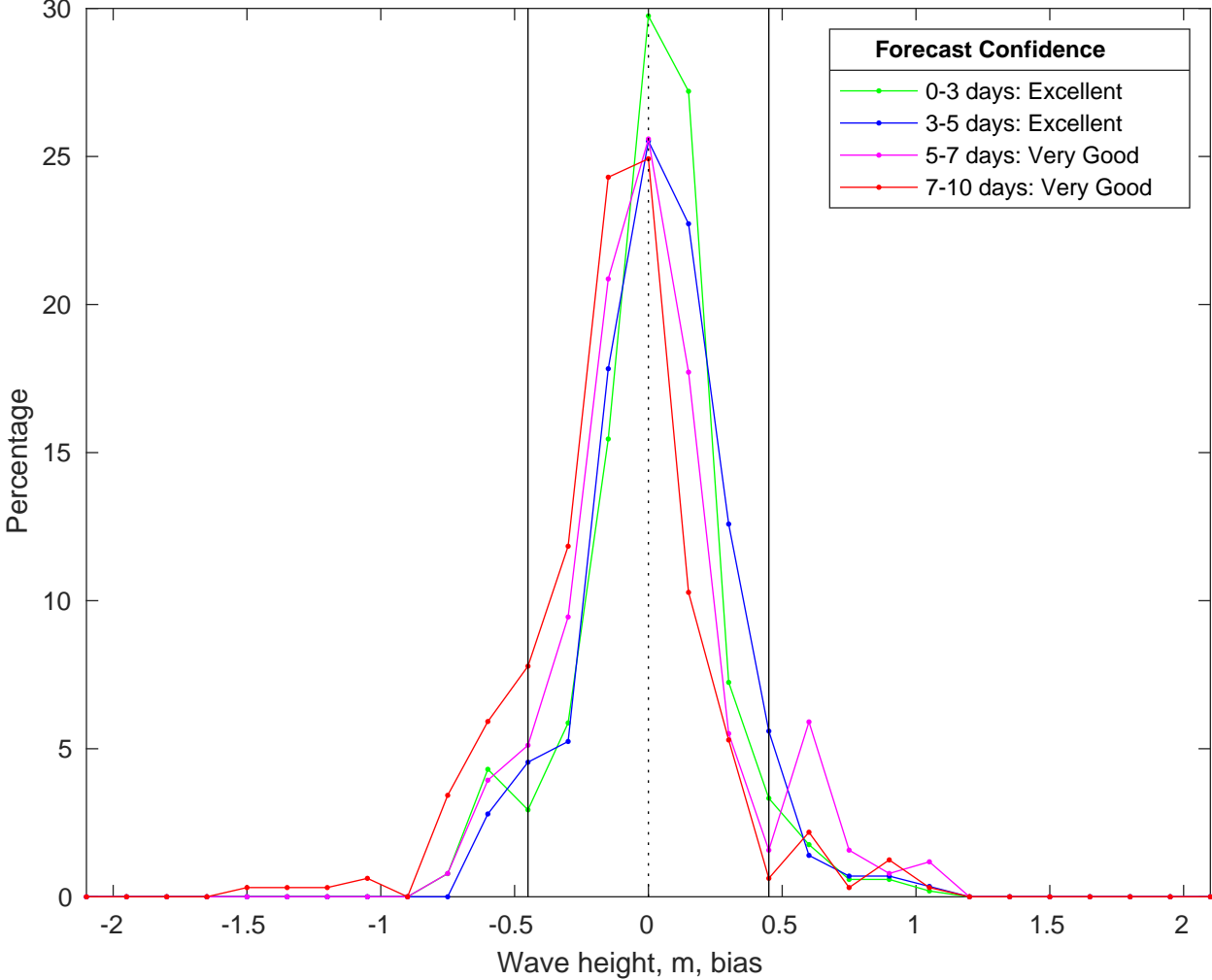
NDBC 46028 vs CMEMS Waves Bias Histogram: 25-Jan-2026
