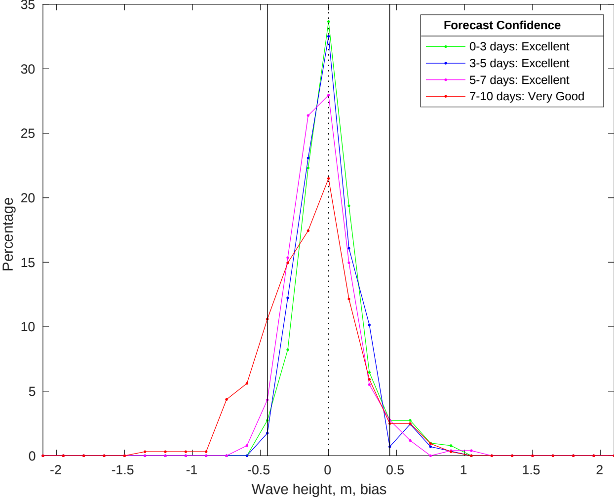
NDBC 46069 vs CMEMS Waves Bias Histogram: 25-Jan-2026
