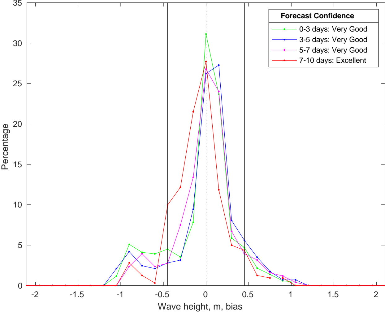
NDBC 46215 vs CMEMS Waves Bias Histogram: 25-Jan-2026
