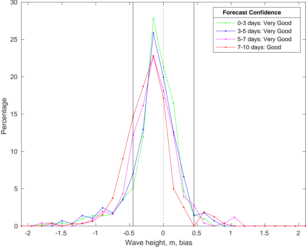
NDBC 46259 vs CMEMS Waves Bias Histogram: 25-Jan-2026
