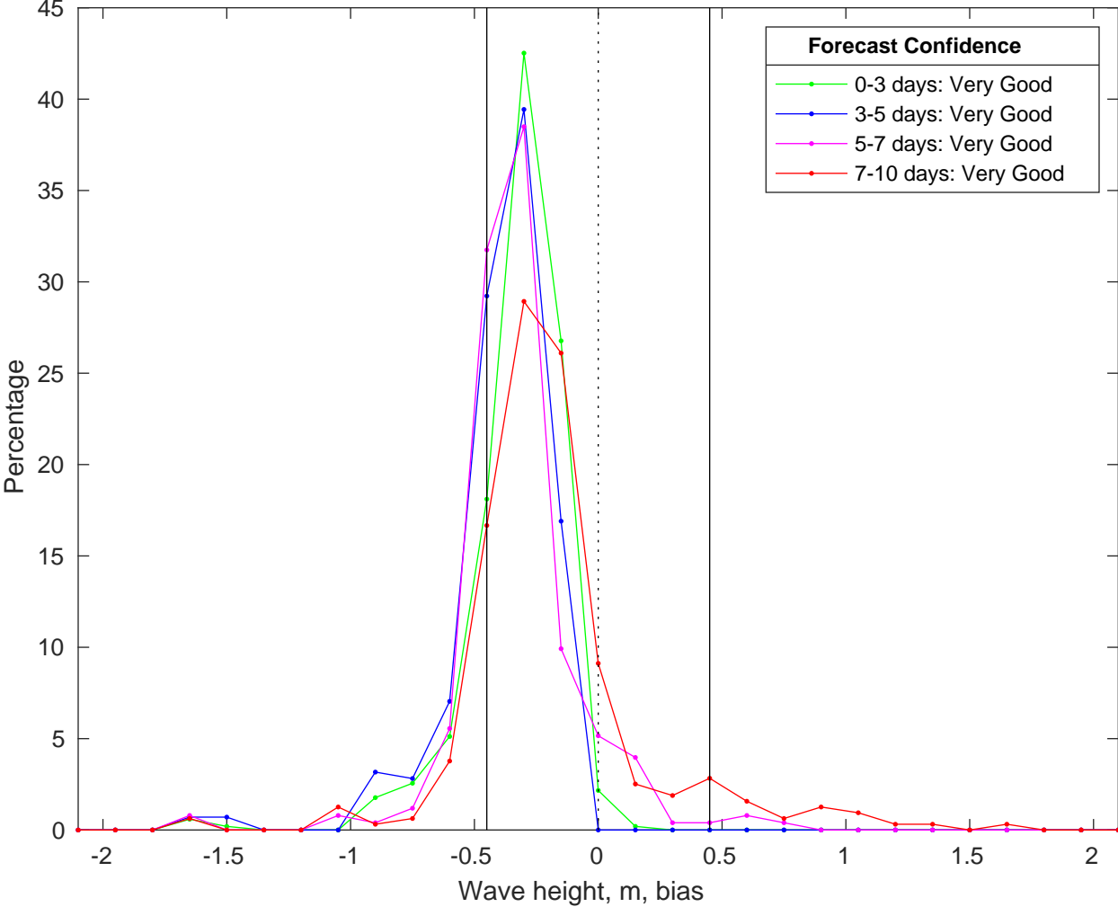
NDBC 51209 vs CMEMS Waves Bias Histogram: 25-Jan-2026
