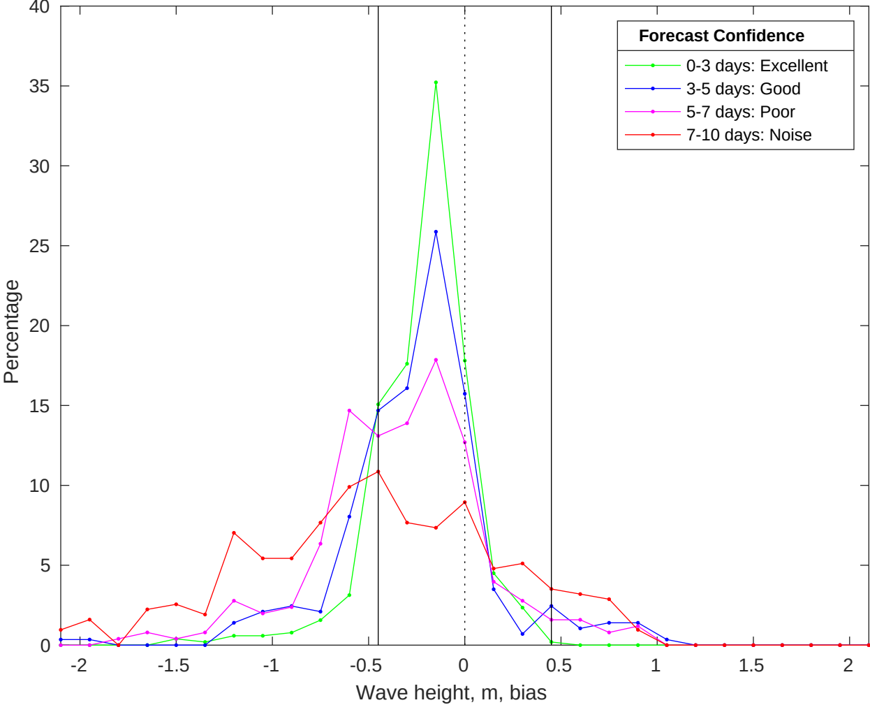
NDBC 42036 vs CMEMS Waves Bias Histogram: 28-Jan-2026
