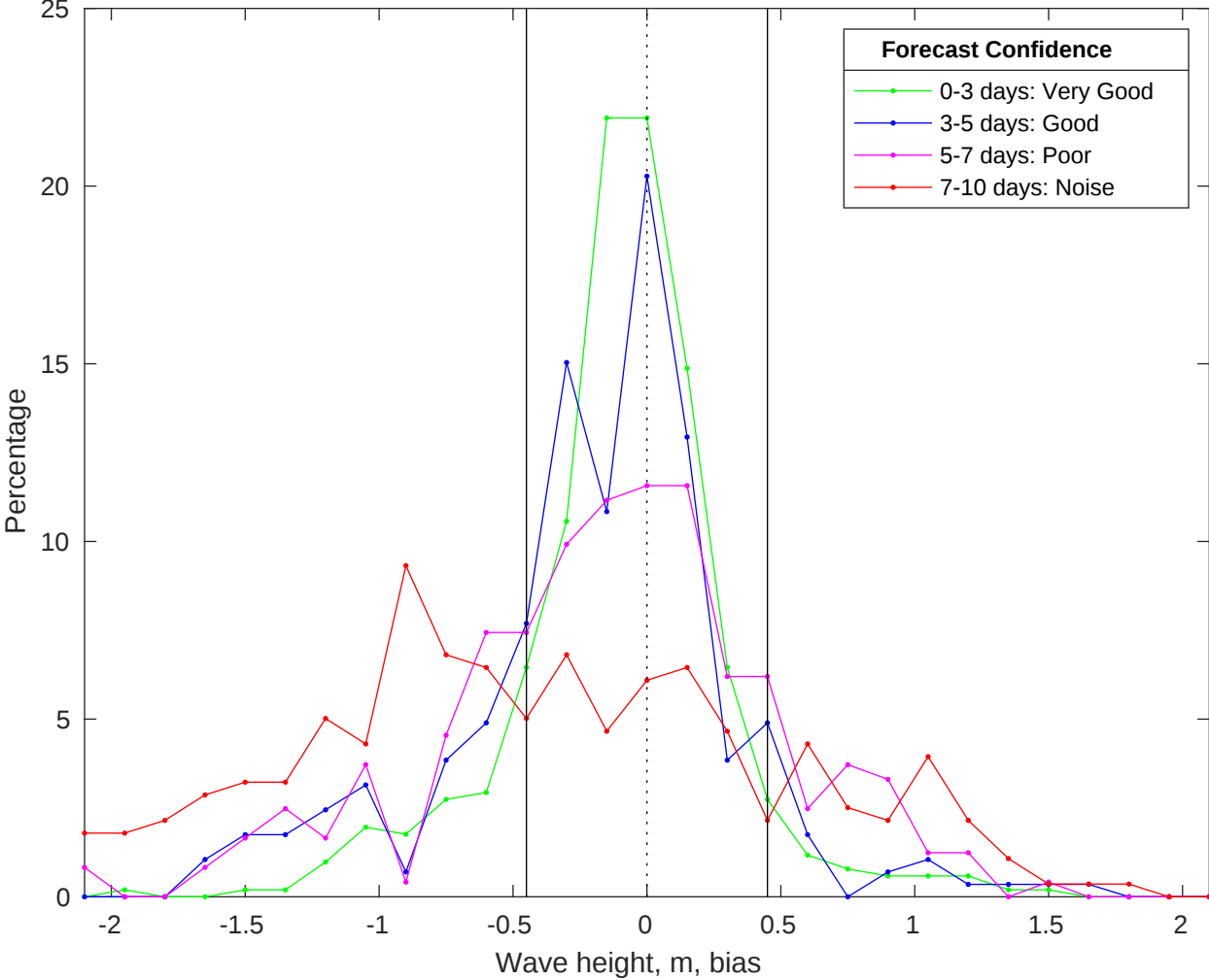
NDBC 44008 vs CMEMS Waves Bias Histogram: 28-Jan-2026
