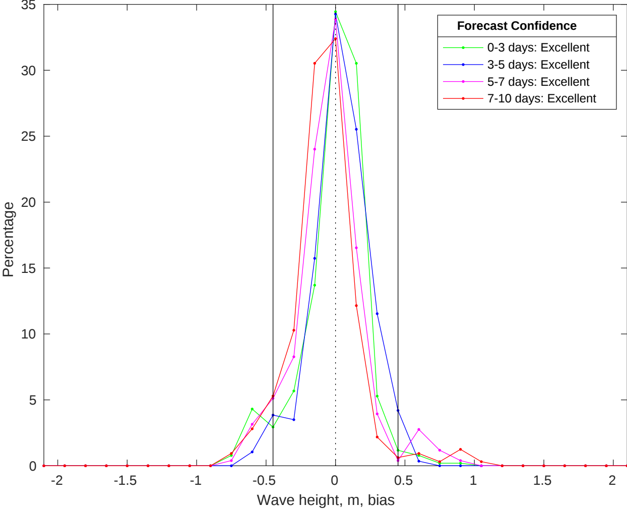
NDBC 46028 vs CMEMS Waves Bias Histogram: 28-Jan-2026
