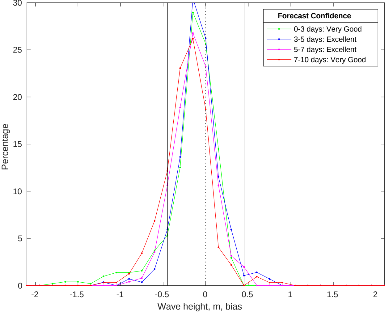
NDBC 46259 vs CMEMS Waves Bias Histogram: 28-Jan-2026
