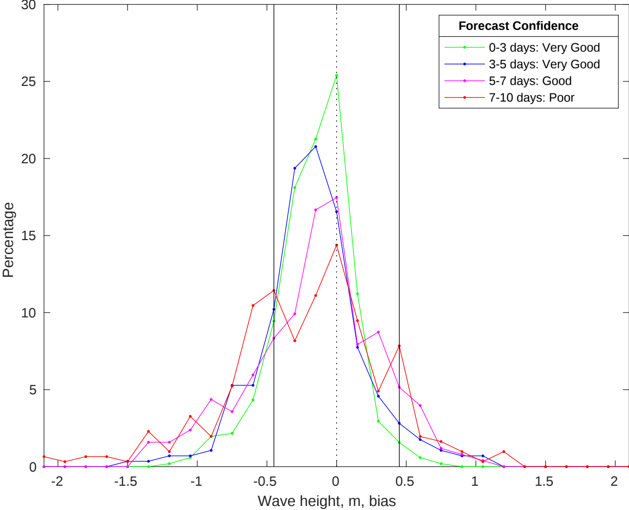
NDBC 41004 vs CMEMS Waves Bias Histogram: 31-Jan-2026
