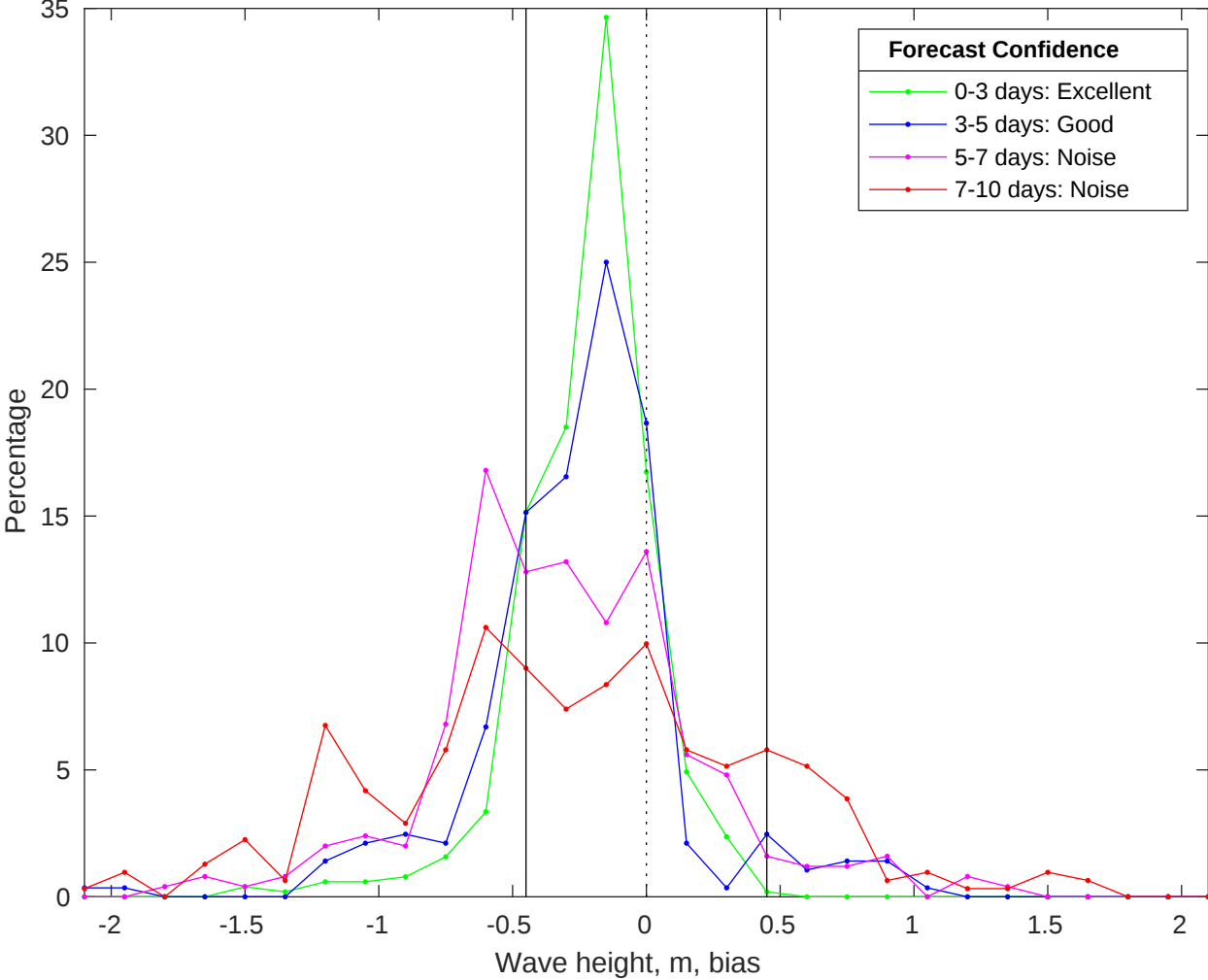
NDBC 42036 vs CMEMS Waves Bias Histogram: 31-Jan-2026
