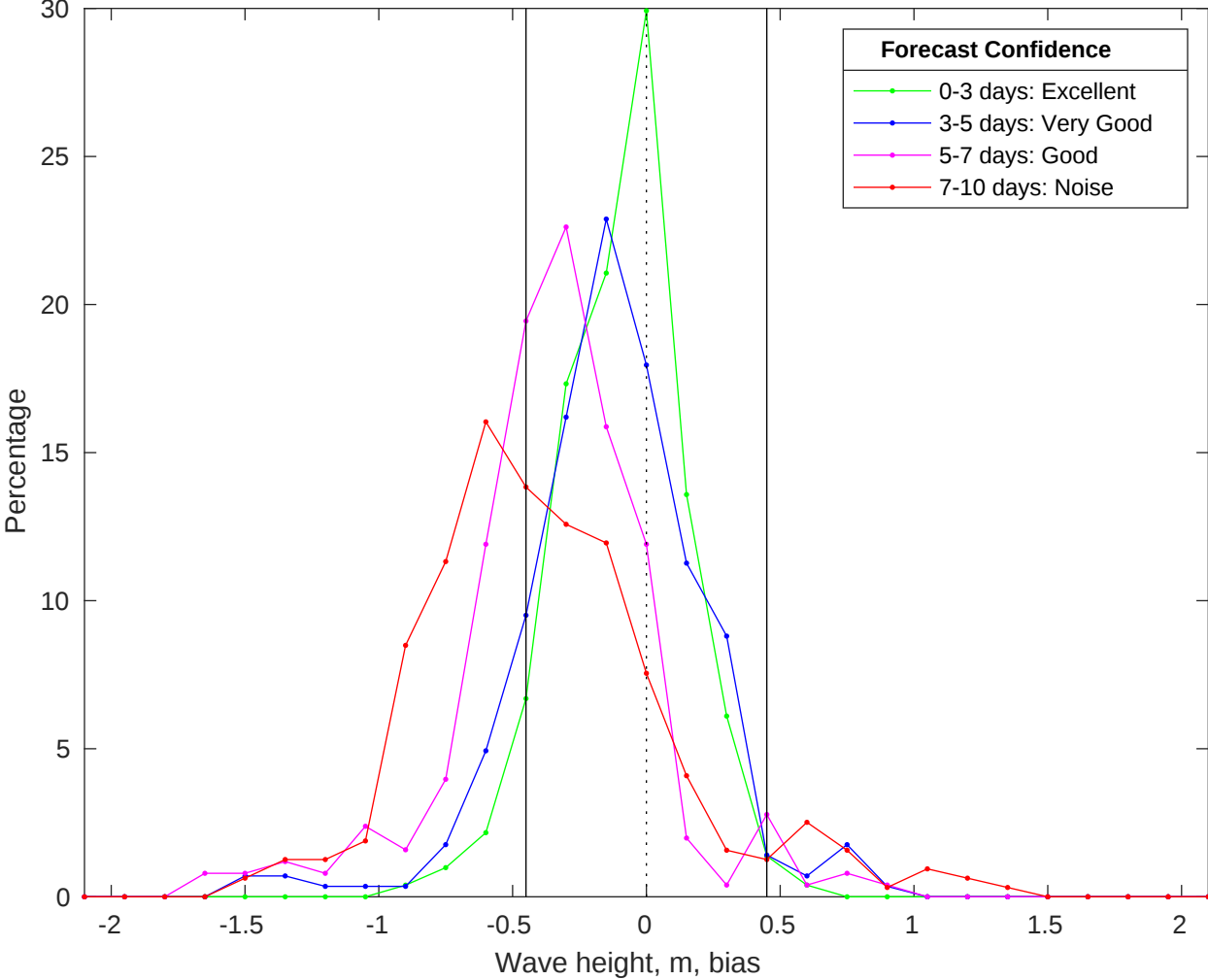
NDBC 46059 vs CMEMS Waves Bias Histogram: 31-Jan-2026
