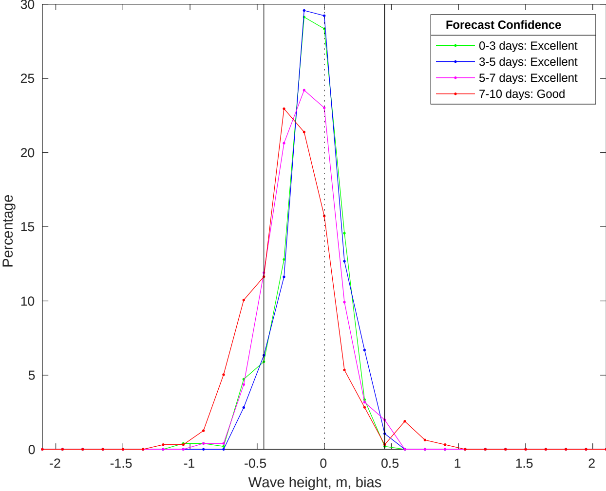
NDBC 46259 vs CMEMS Waves Bias Histogram: 31-Jan-2026
