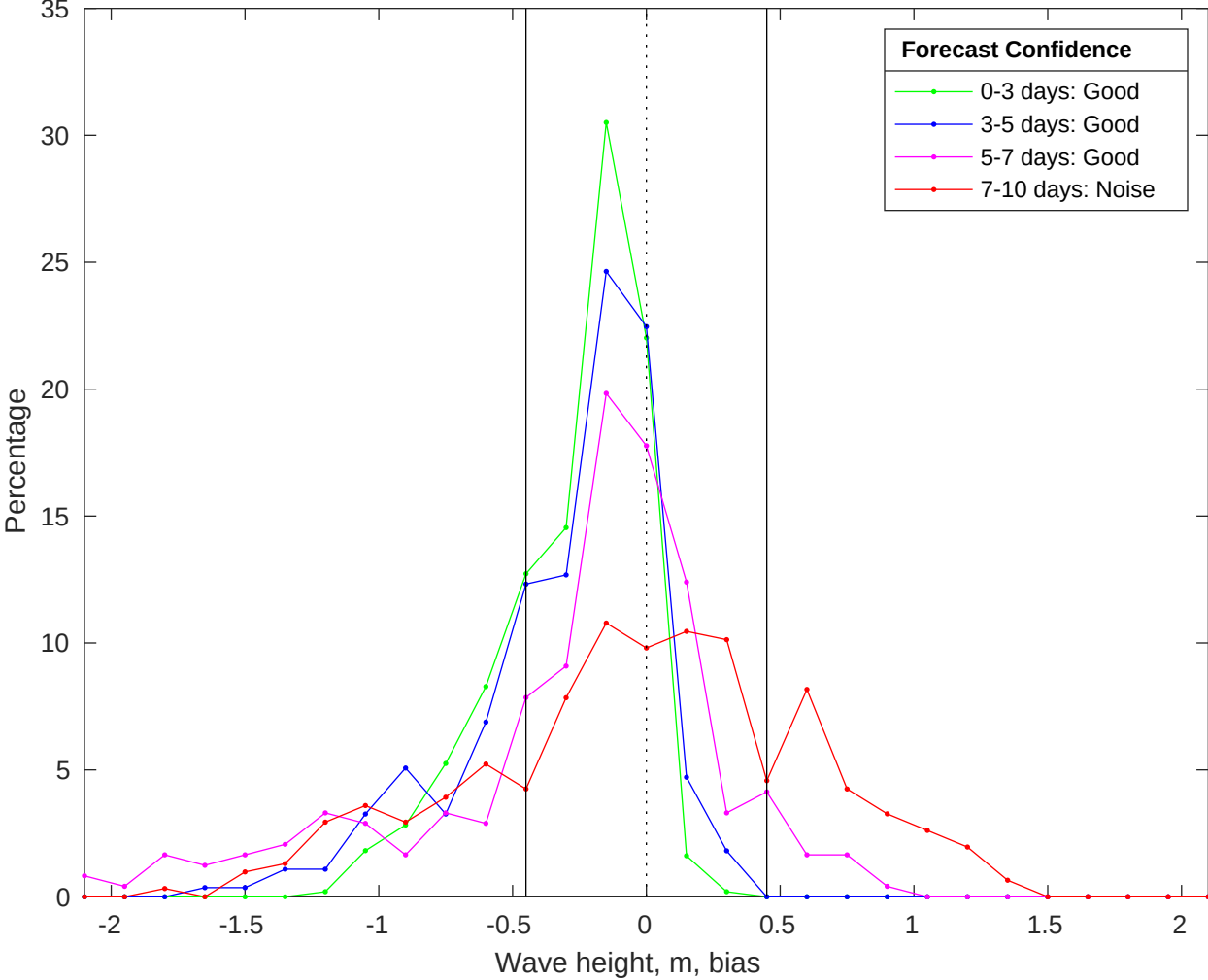
NDBC 42019 vs CMEMS Waves Bias Histogram: 31-Jan-2026
