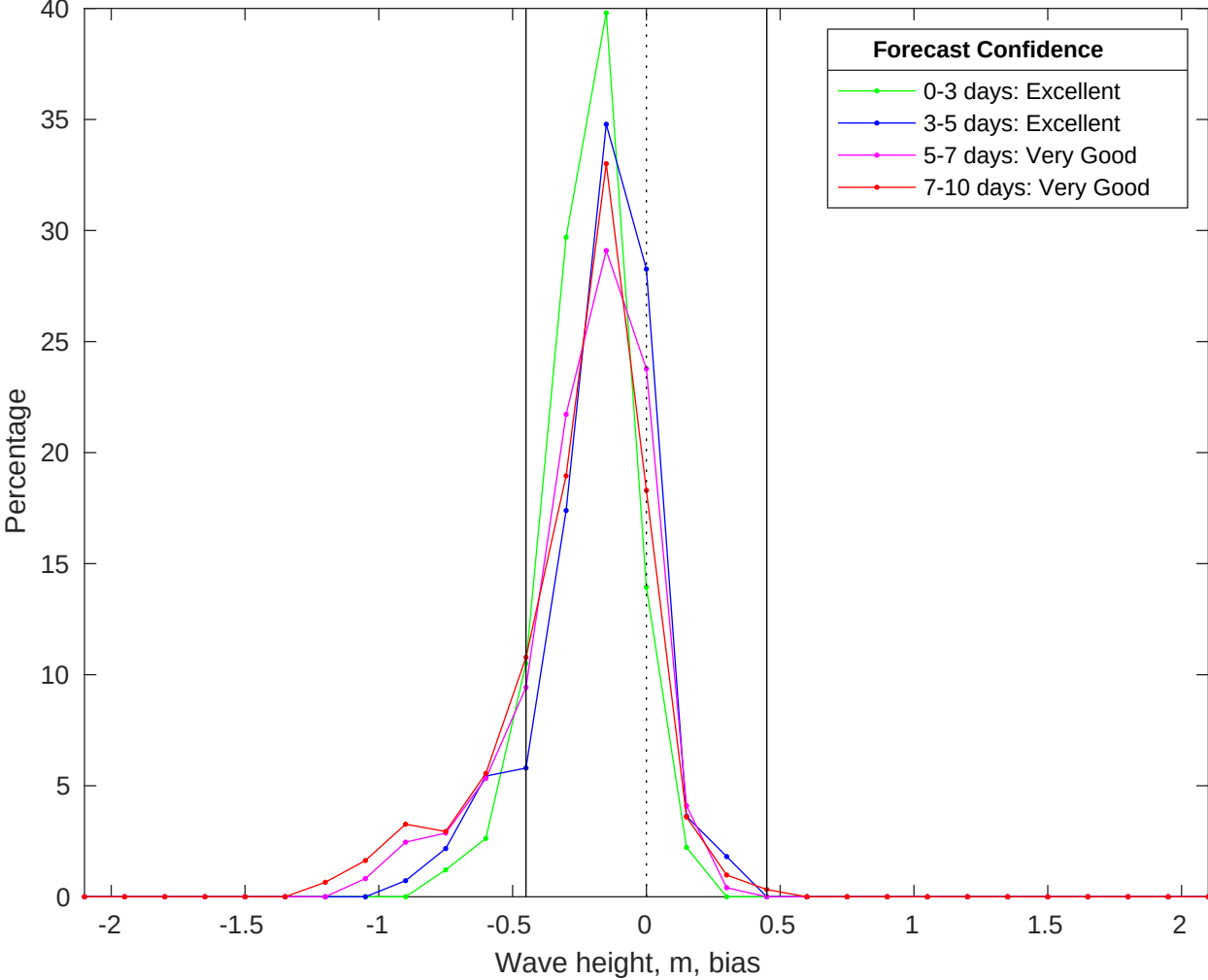
NDBC 52213 vs CMEMS Waves Bias Histogram: 31-Jan-2026
