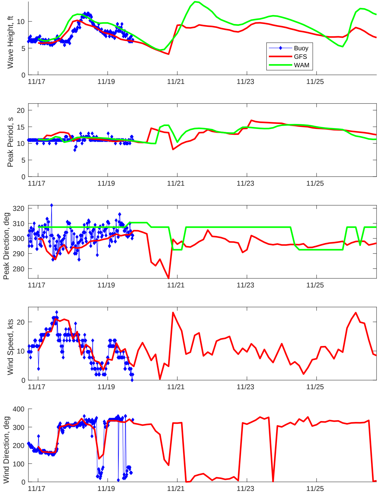
NDBC 46011 : 11/17/25 00:00
