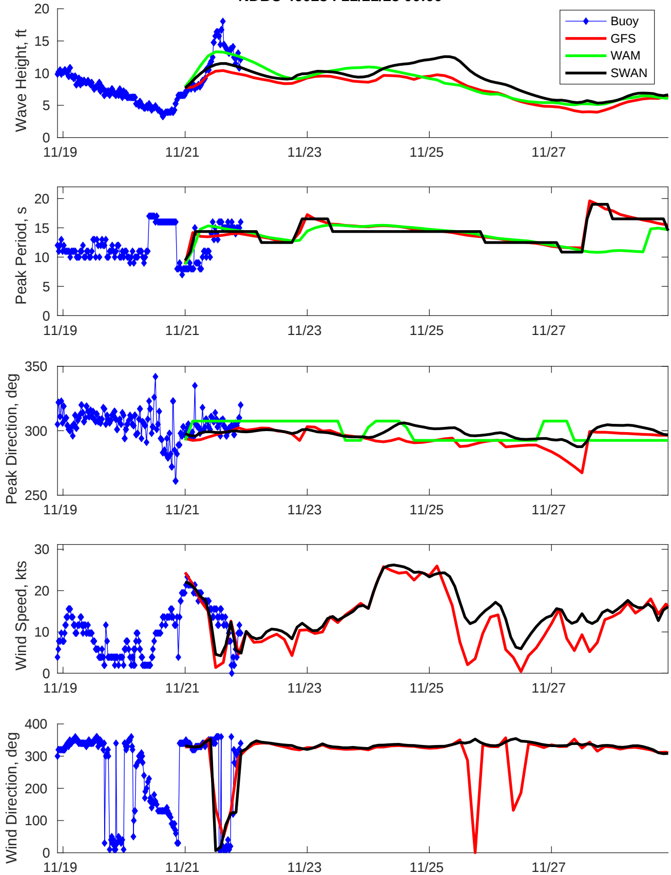
NDBC 46028 : 11/21/25 00:00
