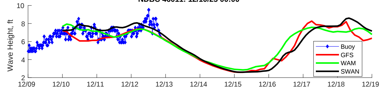
NDBC 46011: 12/10/25 00:00
