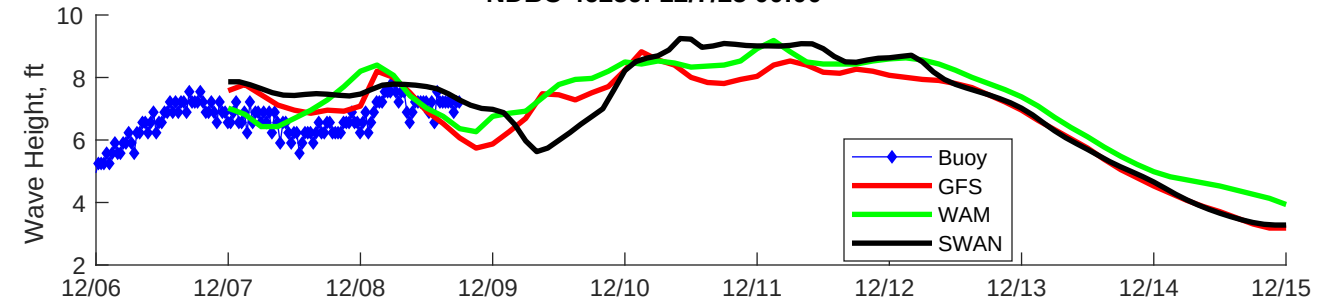
NDBC 46259: 12/7/25 00:00
