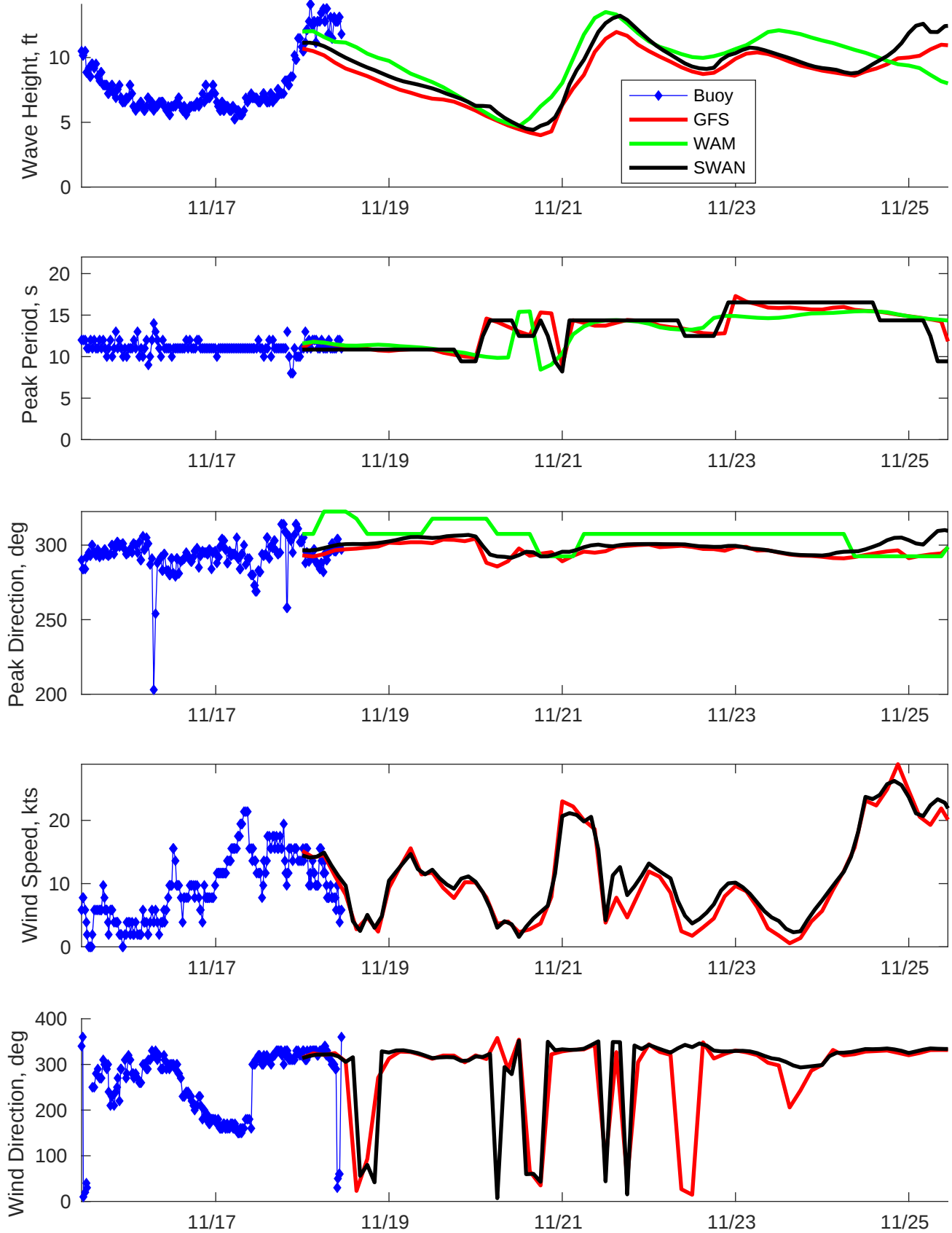
NDBC 46028 : 11/18/25 00:00
