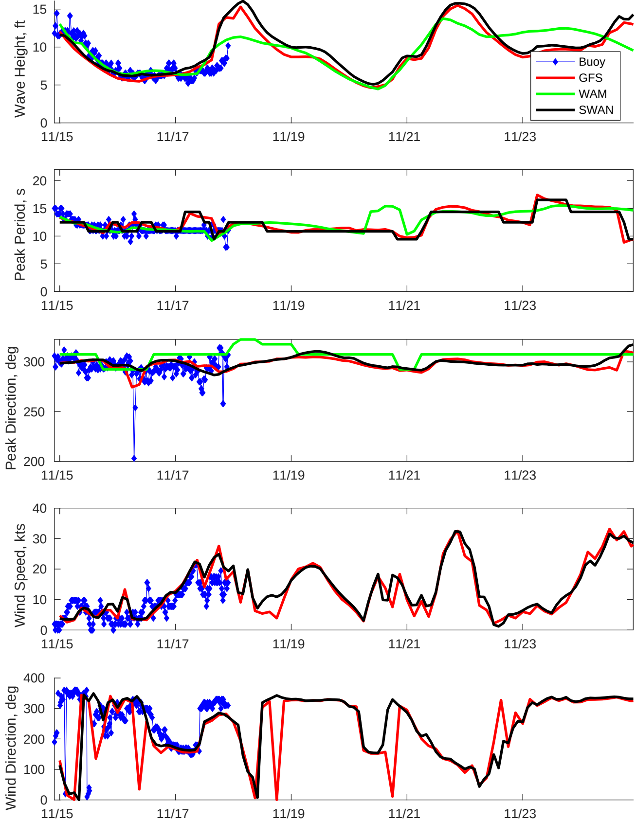
NDBC 46028 : 11/15/25 00:00
