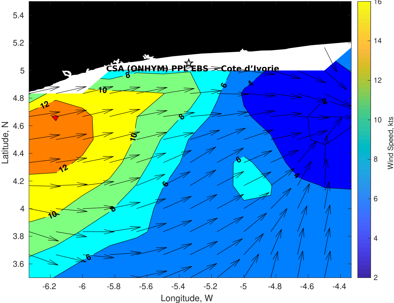
Winds (kts) for CSA (ONHYM) PPL EBS - Cote d'Ivoire at 03-Apr-2025 09:00:00
