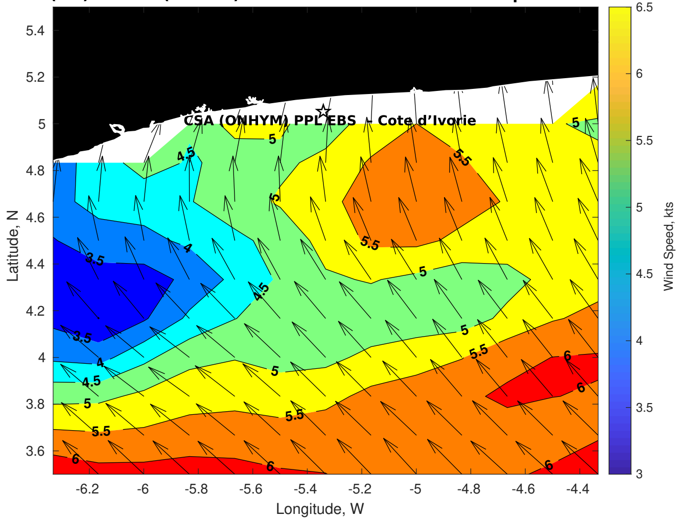
Winds (kts) for CSA (ONHYM) PPL EBS - Cote d'Ivoire at 09-Apr-2025 09:00:00
