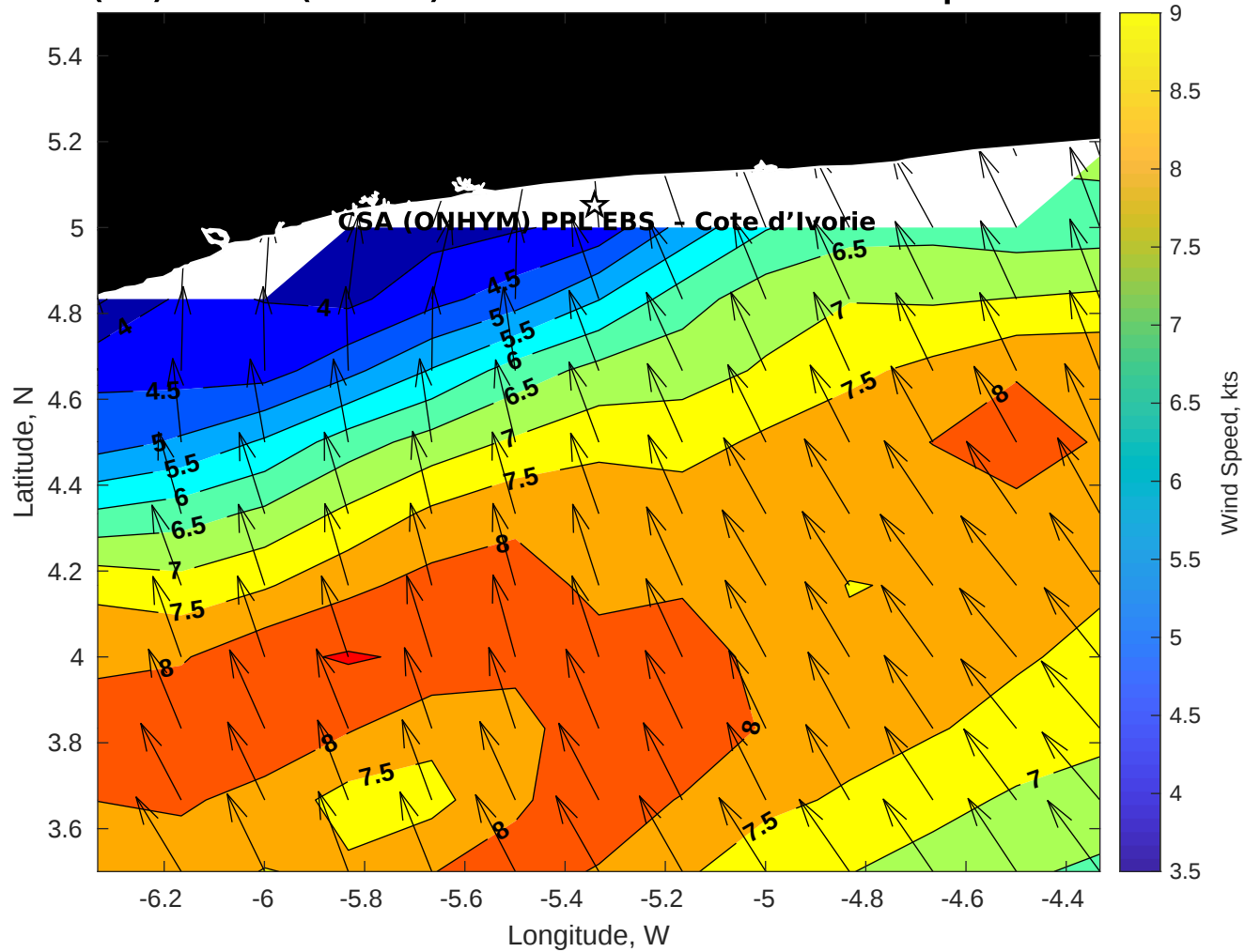
Winds (kts) for CSA (ONHYM) PPL EBS - Cote d'Ivoire at 10-Apr-2025 09:00:00
