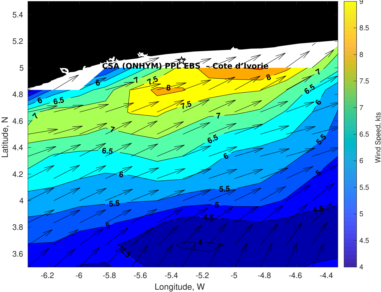
Winds (kts) for CSA (ONHYM) PPL EBS - Cote d'Ivoire at 25-Apr-2025 09:00:00
