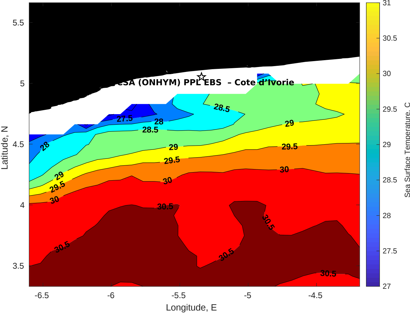
SST for CSA (ONHYM) PPL EBS - Cote d'Ivoire at 25-Apr-2025 00:00:00
