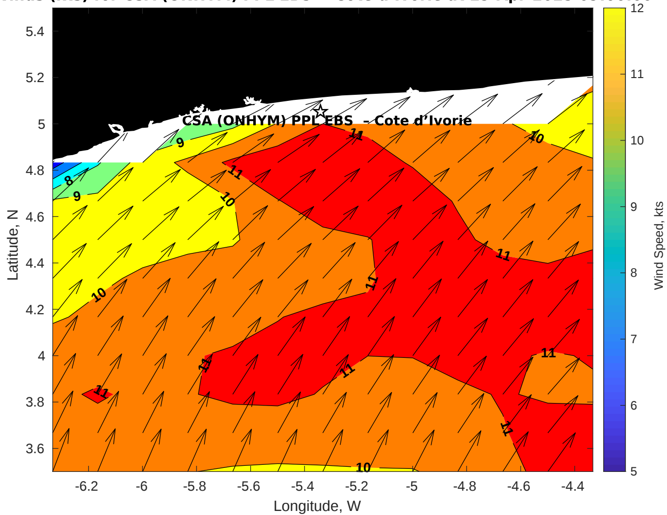
Winds (kts) for CSA (ONHYM) PPL EBS - Cote d'Ivoire at 29-Apr-2025 09:00:00
