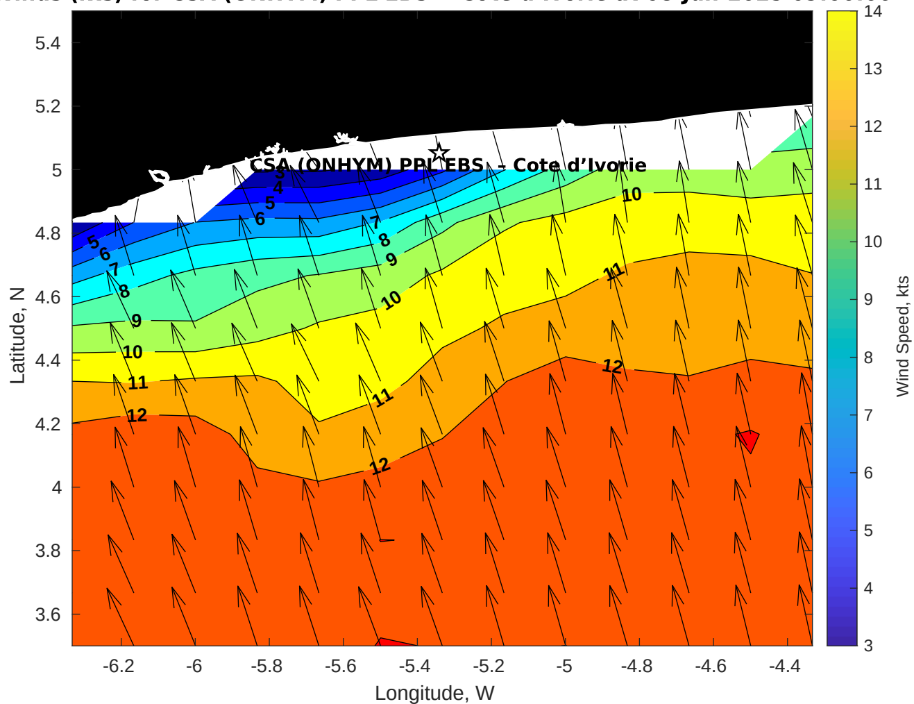
Winds (kts) for CSA (ONHYM) PPL EBS - Cote d'Ivoire at 08-Jun-2025 09:00:00
